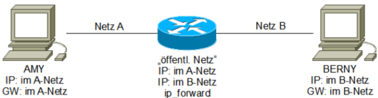
Abbildung 1: VPN: End-to-End im Transport-Modus (manuell konfiguriert)
